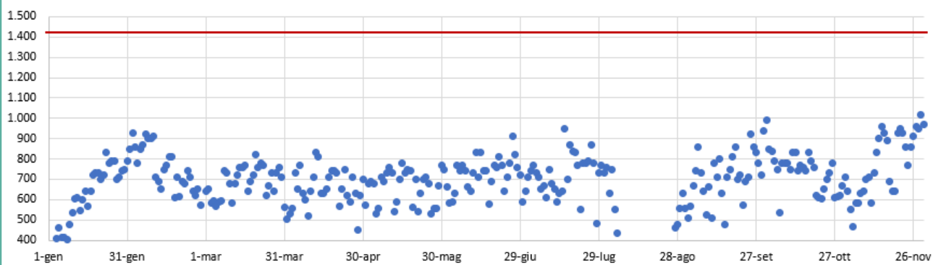
SOLFATI (mg/l)
